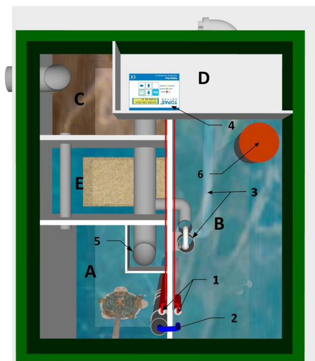
Figur 1: Grundplan för TOPAS Plus 10
