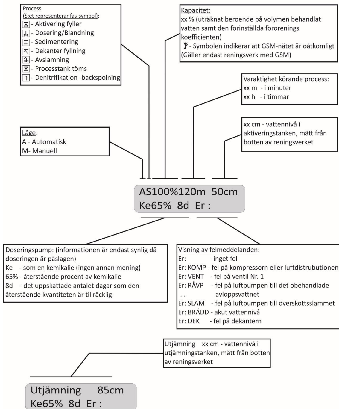
Figur 5: Topas Plus Displayträd
