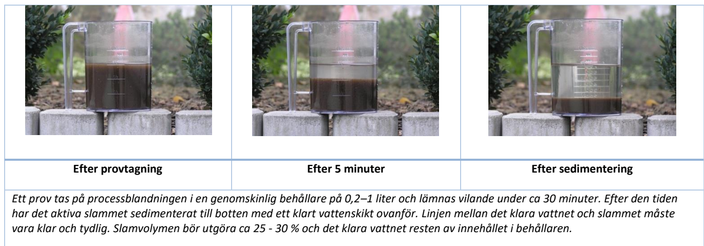
Figur 2: Kontroll av slammängden i processtanken
