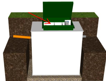
Topas Plus 10-80 utan grovrenstank
