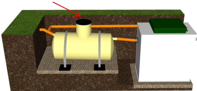
Topas Plus 10-80 med Grovrenstank
